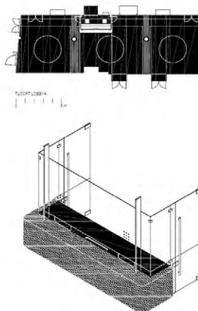
Rekonstrukcija biljetarnice kina Valli u Puli
